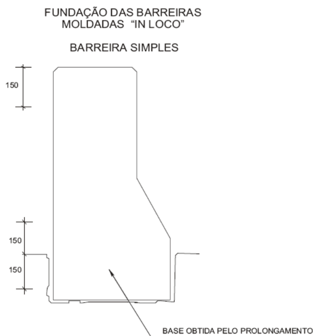
Figura 04 - Fundação
