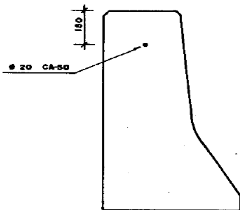
Figura 02 – Barreira moldada “in loco”
